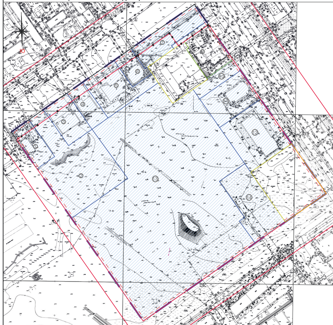
Чертеж межевание территории
