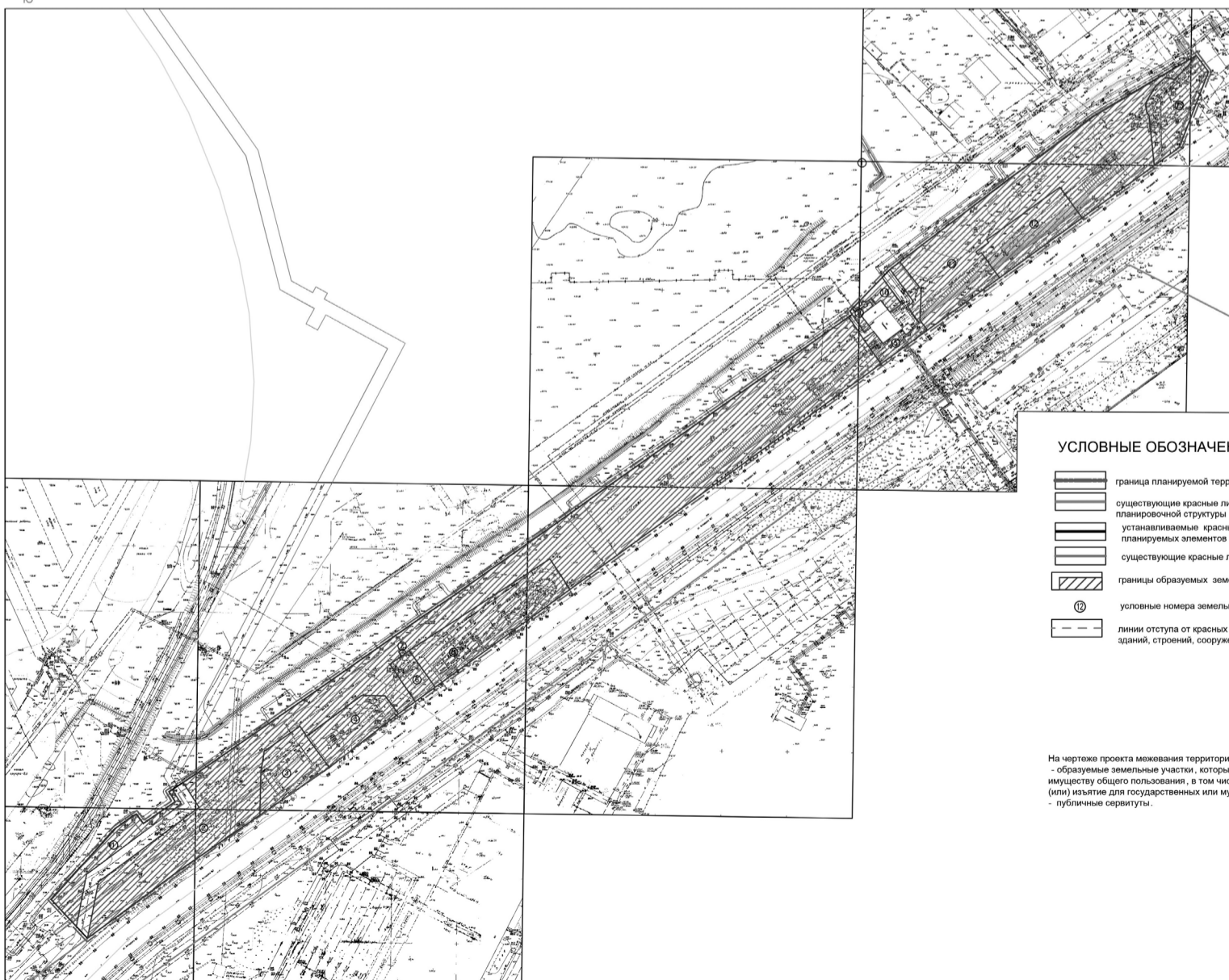
Чертеж межевания территории. М 1:2000
